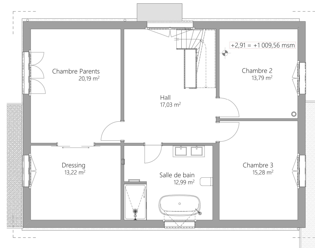
Etage
