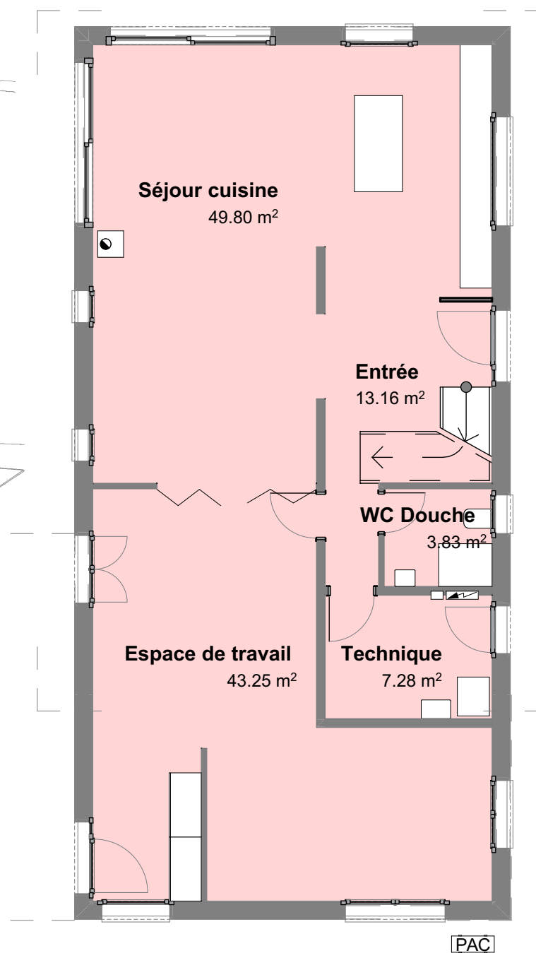
Rez-de-chaussée
